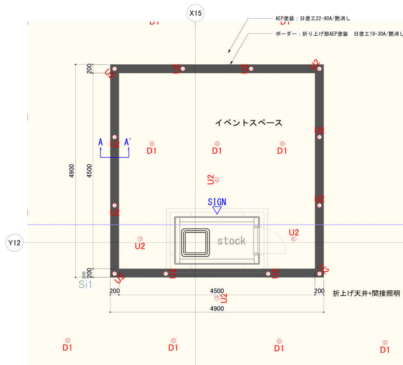
天井伏図
